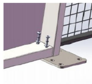
3 Poutre basse M10*65
