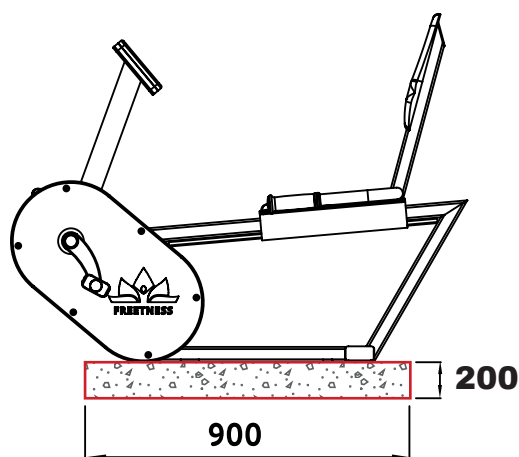
VUE LATÉRALE
