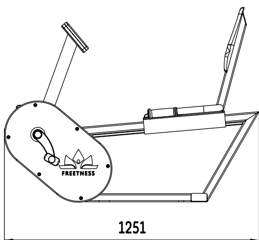
Vue latérale
