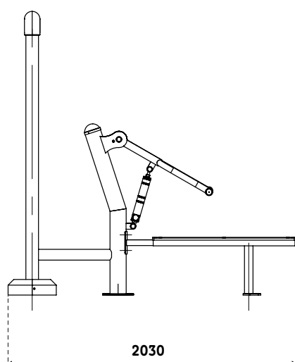
Vue latérale
