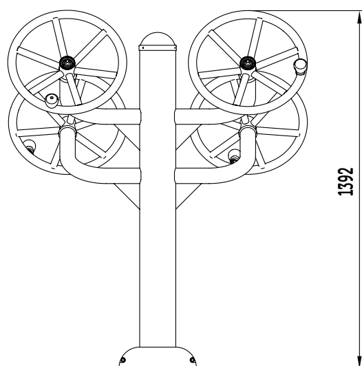
Vue latérale
