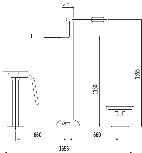
Vue latérale
